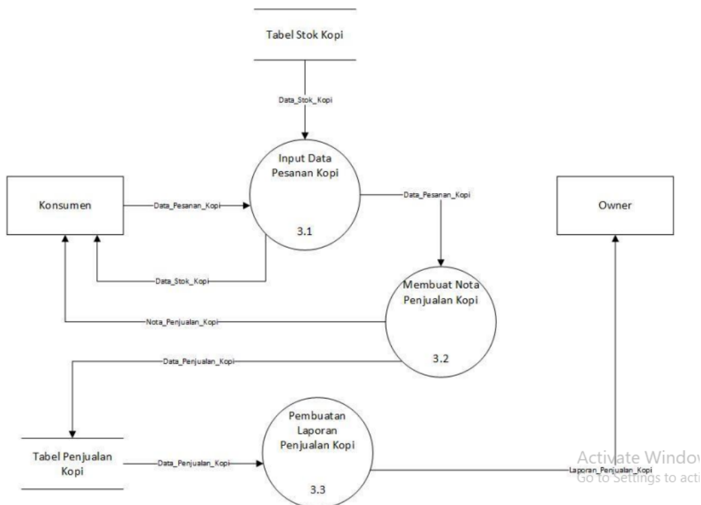
Sistem informasi akuntansi pada penjualan
