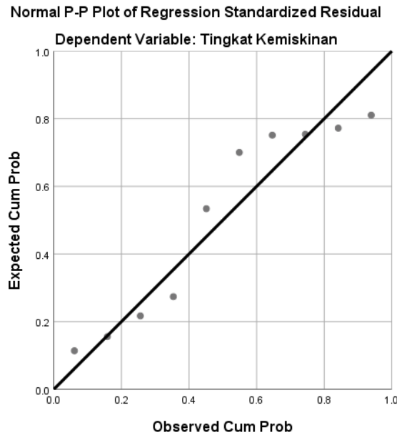
Uji Multikolinieritas
